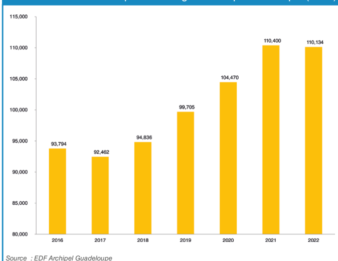
Production d'électricité à partir d'énergie solaire photovoltaïque (GWh)
