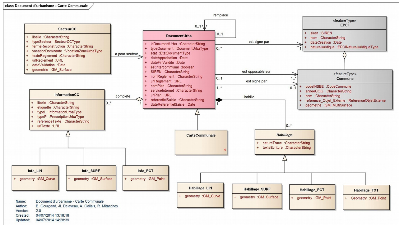
Les différentes classes et leurs relations représentées en UML
